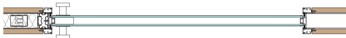
Puerta corredera Flat D00R - DU010 con hoja de 2 vidrio enmarcados Porta corrediça Flat D00R - DU010 com folha de 2 vidros encaixilhados Sliding door, Flat D00R - DU010 with double-glazed leaf, alum. frame Porte coulissante Flat D00R - DU010 avec panneau de double vitrage
