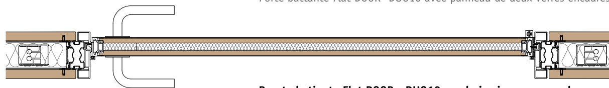
Puerta batiente Flat D00R - DU010 con hoja ciega enmarcada Porta batente Flat D00R - DU010 com folha cega encaixilhada Hinged door, Flat D00R - DU010 with blank leaf, aluminium framed Porte battante Flat D00R - DU010 avec panneau melaminé encadré
