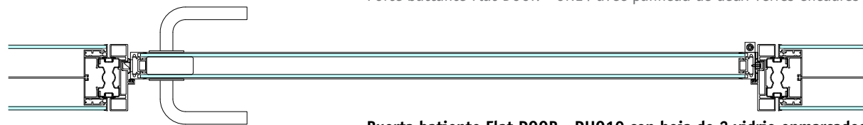
Puerta batiente Flat D00R - DU010 con hoja de 2 vidrio enmarcados Porta batente Flat D00R - DU010 com folha de 2 vidros encaixilhados Hinged door, Flat D00R - DU010 with double-glazed leaf, alum. framed Porte battante Flat D00R - DU010 avec panneau de deux verres encadrés
