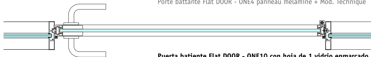
Puerta batiente Flat D00R - ONE10 con hoja de 1 vidrio enmarcado Porta batente Flat D00R - ONE10 com folha de 1 vidro encaixilhado Hinged door, Flat D00R - ONE10 with a single glass leaf, alum. framed Porte battante Flat D00R - ONE10 avec panneau d'un verre encadré
