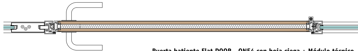
Puerta batiente Flat D00R - ONE4 con hoja ciega + Módulo técnico Porta batente Flat D00R - ONE4 com folha cega + Módulo técnico Hinged door, Flat D00R - ONE4 with blank leaf + Technical compartment Porte battante Flat D00R - ONE4 panneau melaminé + Mod. Technique
