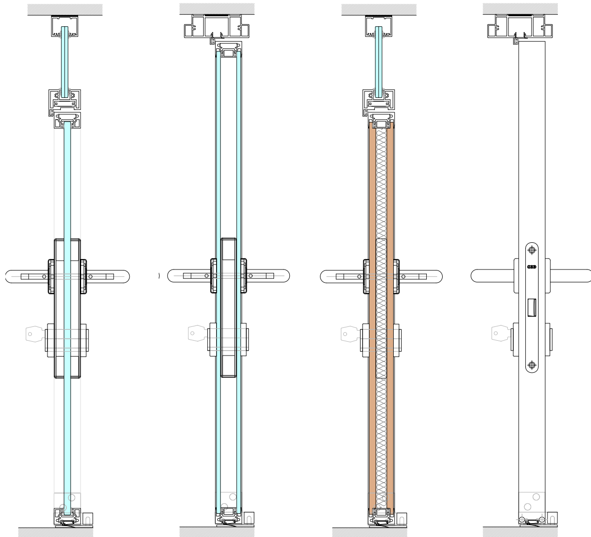
Sección vertical / Seção vertical / Vertical View / Section Verticale
