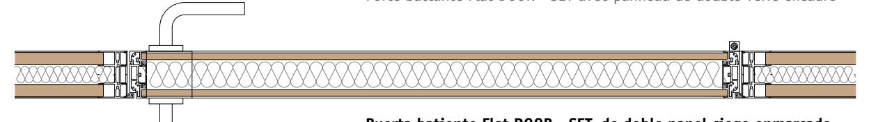
Puerta batiente Flat D00R - SET, de doble panel ciego enmarcado Porta batente Flat D00R - SET de painel cego duplo encaixilhado Hinged door, Flat D00R - SET double solid panel aluminium framed leaf Porte battante Flat D00R - SET avec panneau plein double encadré
