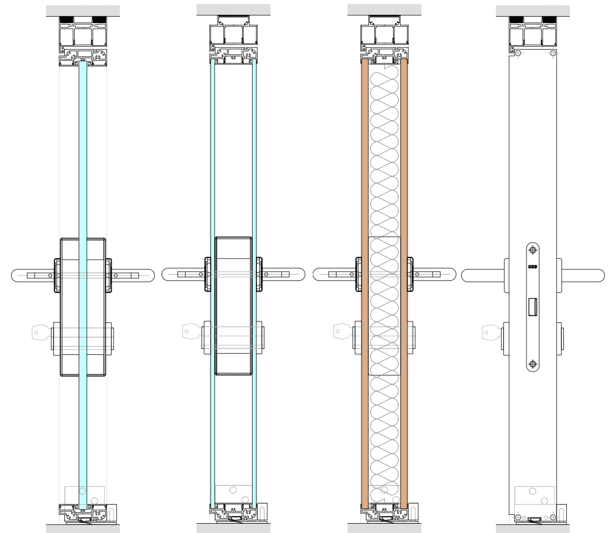
Sección vertical / Seção vertical / Vertical View / Section Verticale
